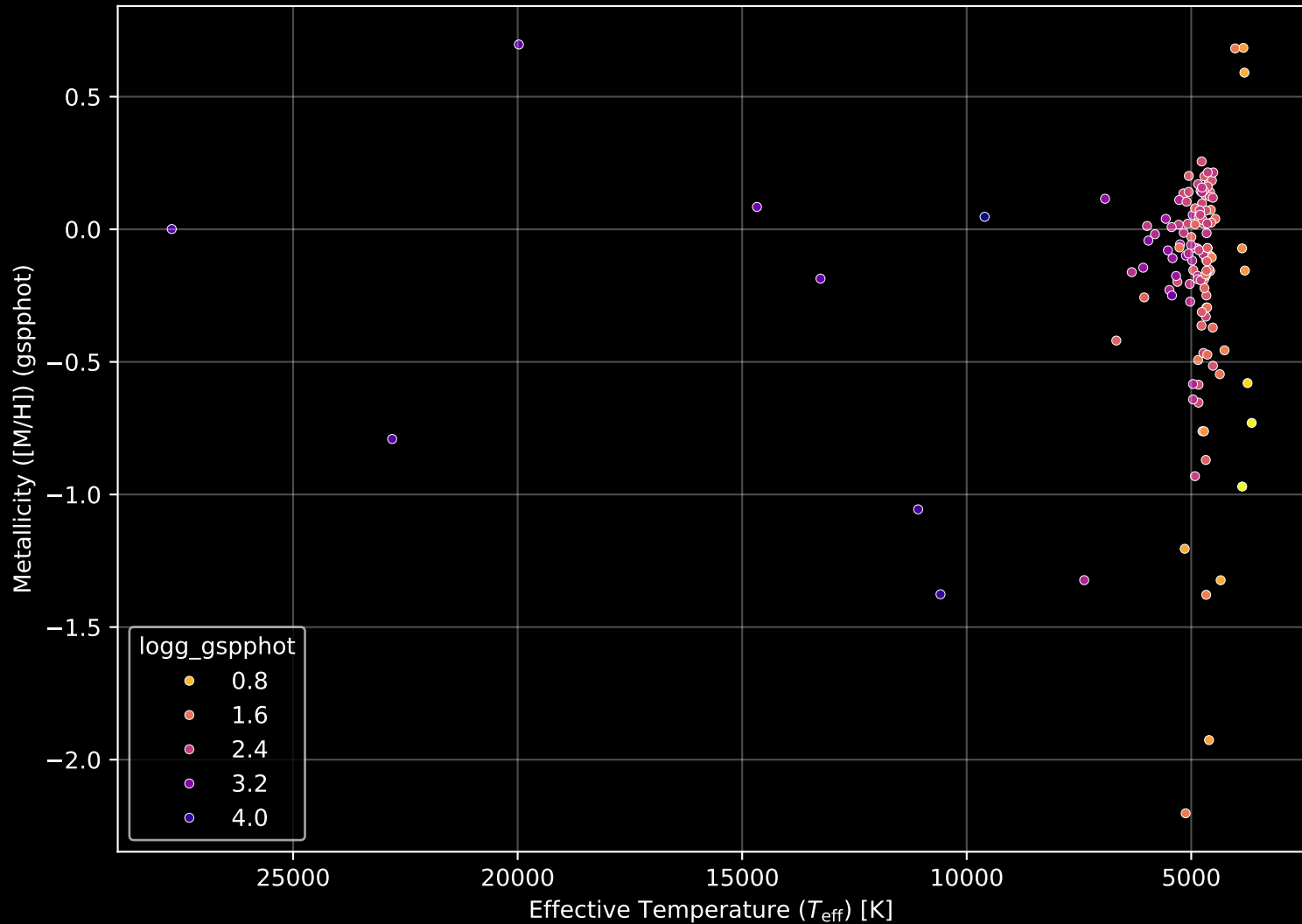
APOGEE DR17 Field: [Cas_S] Stellar Population Parameters (n= 131)
